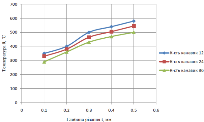
Рис. 4. Залежність температури різання від глибини різання при V_{\text{д}}=10\text{м/хв} , V_{\text{кд}}=35\text{м/с} , t=0.05\text{ мм}
