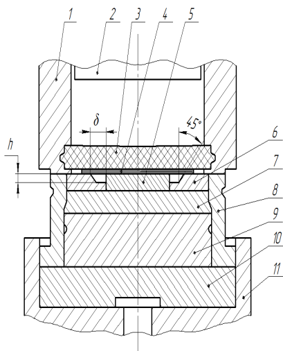
Рис. 1 – Технологічна схема вирубання поліуретаном із застосуванням матриць і опорних рамок: 1 – ствол машини; 2– бойок, 3– діафрагма поліуретанова; 4 – заготовка; 5 – матриця; 6 – опорна рамка; 7 – диск; 8– обойма; 9,10 – плита; 11 – контейнер.
