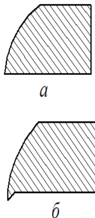
Рис. 4 – Приклади зрізу деталей: а – пластичних матеріалів, б – малопластичних матеріалів.
