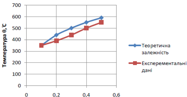
Рис. 2. Вплив глибини різання на температуру при V_s = 10 м/хв, V_{kp} = 35 м/с, \varepsilon = 12
