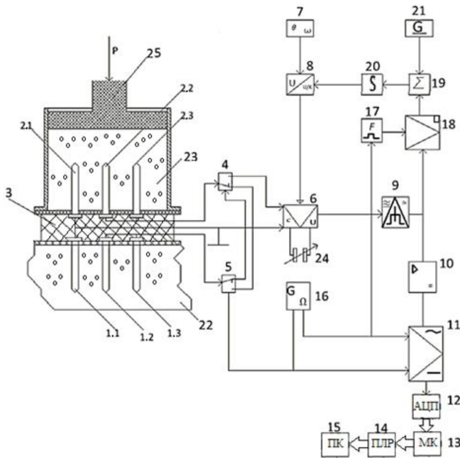
Рис. 1. Структурна схема вимірювальної системи вологості зерна
