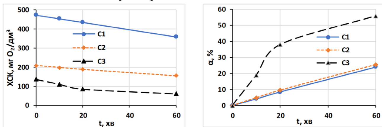
Рис. 2. Кінетика зміни ХСК та ступеня окиснення розчинів амоксициліну з початковими концентраціями: C_1 = 288 мг/дм 3 ; C_2 = 144 мг/дм 3 ; C_3 = 72 мг/дм 3
