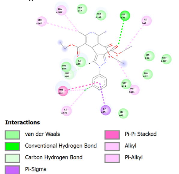
Рис. 1d. Сполука 4c , InhA (PDB id: 4TRN) docking score -7.1 ккал/моль
