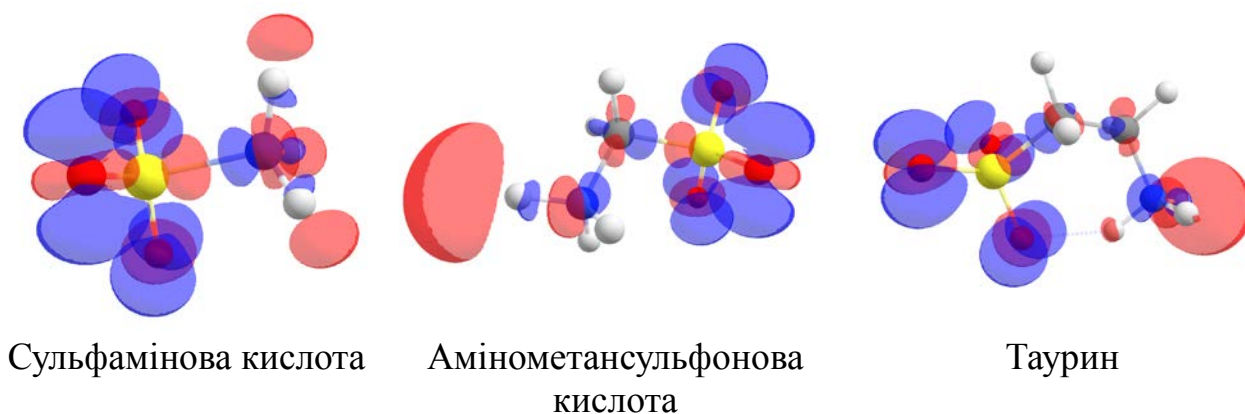
Рис. 1. Графіки конденсованого подвійного дескриптора (CDD) для молекул. Червоні ділянки відповідають нуклеофільним центрам (де CDD від’ємний), а сині ділянки — електрофільним центрам (де CDD додатний).
