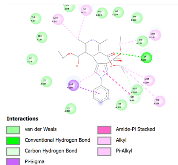
Рис. 1b. Сполука 4a , InhA (PDB id: 4TRN) docking score -7.0 ккал/моль
