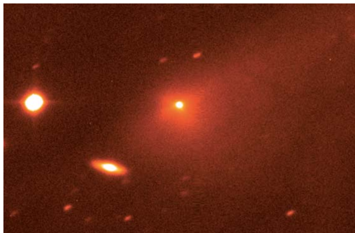
Снимок кометы 67P/Чурюмова-Герасименко, полученный 26 января 2004 г. (комета в центре снимка).
