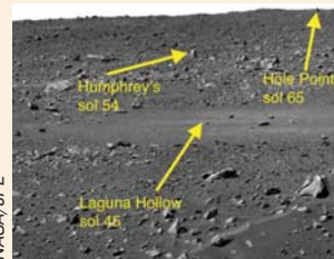
На изображении, полученном навигационной камерой Spirit, показаны места трех остановок марсохода в кратере Гусева. В низине Laguna Hollow (Лагуна пустоты) одним из своих колес Spirit вырыл ямку и осмотрел ее. Следующая остановка была сделана для исследования камня Humphrey . Далее Spirit отправился к камню, который называли Hole Point , в сторону кратера Bonneville .
