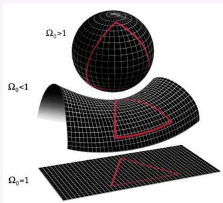
Иллюстрация замкнутого, разомкнутого и плоского пространства Вселенной, если масса всего вещества, содержащегося в ней, больше, меньше или равна критической, соответственно.
