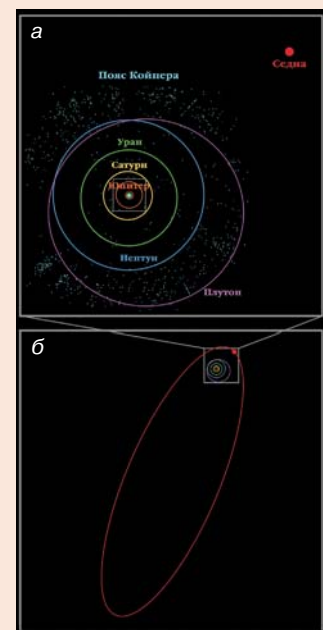
Орбита 2003 VB16 (Sedna) в Солнечной системе. а — сегодняшнее положение Седны относительно внешних планет, б — орбита Седны.
