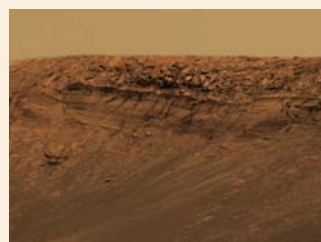
Участок кратера Endurance, называемый утесом Бернса (Burns Cliff). Исследование этого утеса может дать ключ к пониманию геологического прошлого Марса.
