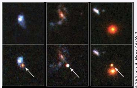
Это снимки самых удаленных от нас вспышек Сверхновых, зарегистрированных космическим телескопом им. Хаббла. Они настолько яркие, что могут наблюдаться с огромных расстояний через несколько миллиардов лет. Это позволяет астрономам определять темп расширения Вселенной и гравитационное влияние "темной материи", наполняющей пространство.
