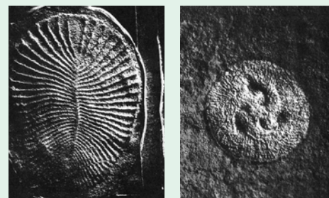
Слева: отпечаток двустороннесимметричного организма с характерной для вендской фауны "симметрией скользящего отражения" — сегментацией, не типичной для фанерозойской фауны, при которой идентичные элементы правой и левой сторон тела сдвинуты друг относительно друга. Для современного зоолога это удивительная симметрия выглядит как явление из другого мира. Справа: отпечаток медузоида с трехлучевой симметрией тела, не встречающейся у фанерозойских животных.
