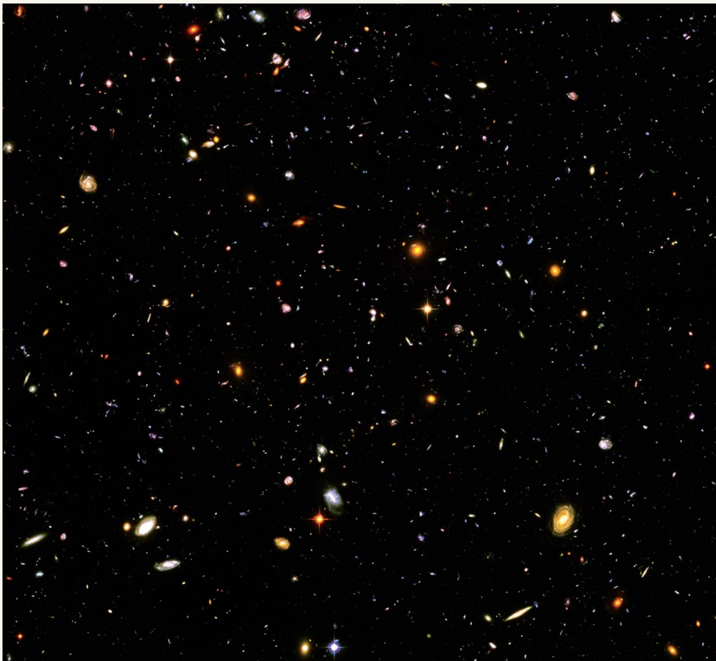
NASA, ESA, S. Beckwith (STScI) and the HUDF Team
