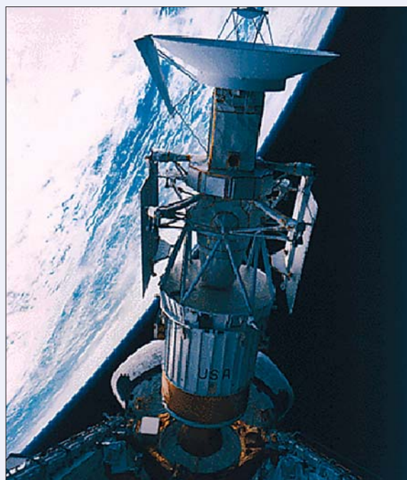
Извлечение Magellan из грузового отсека Atlantis.
