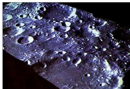
Первые изображения, переданные КА Чанъэ-1: цифровой снимок поверхности (слева), цветная топографическая диаграмма (справа)
