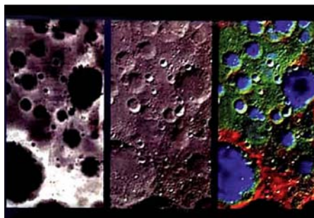
Первые изображения, переданные КА Чанъэ-1: цифровой снимок поверхности (слева), цветная топографическая диаграмма (справа)
