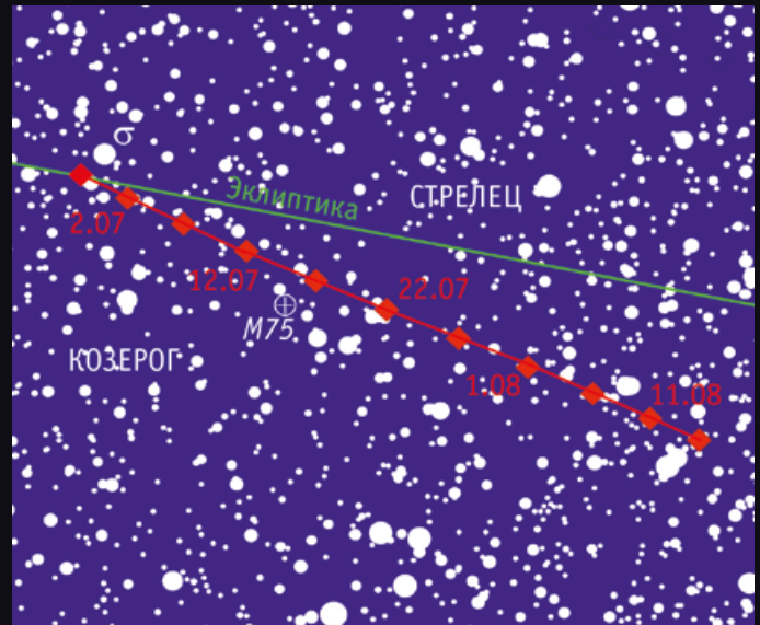
Видимый путь астероида Флора (8 Flora) в июле-августе 2013
