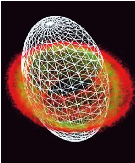
▲ На этом рисунке приведена трехмерная модель туманности «Кольцо», созданная на основе анализа последних наблюдений телескопа Hubble. Красный цвет соответствует свечению главного кольца, вызванного излучением ионизированного азота. Зеленый цвет относится к эмиссии кислорода – главного компонента кольца. Окружность вокруг 3D-модели демонстрирует структуры, долгое время остававшиеся недоступными взгляду астрономов.
