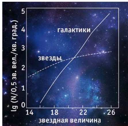
▲ Количество звезд и галактик на квадратный градус неба в интервале 0,5 звездной величины в зависимости от их блеска в голубой области спектра.
