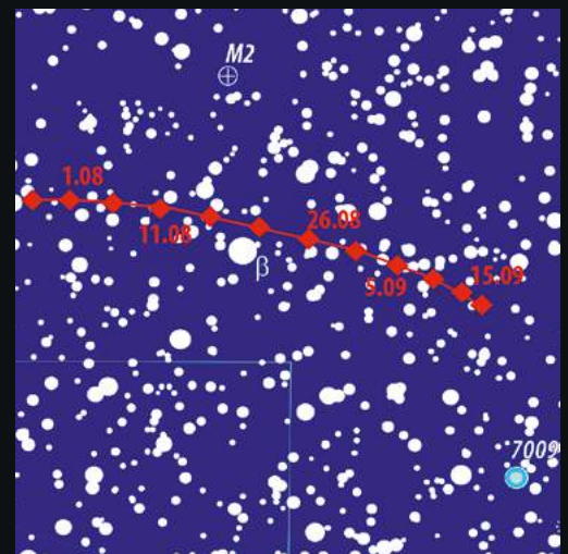
Видимый путь астероида Ирида (7 Iris) по созвездиям Водолея в августе-сентябре 2013 г.
