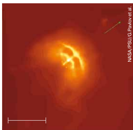
▲ Плерион пульсара Vela.
