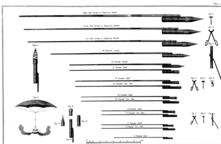
▲ Британский инженер Уильям Конгрив (Sir William Congreve) успешно использовал ракеты в войне с Наполеоном. Рисунок 1814 г.
