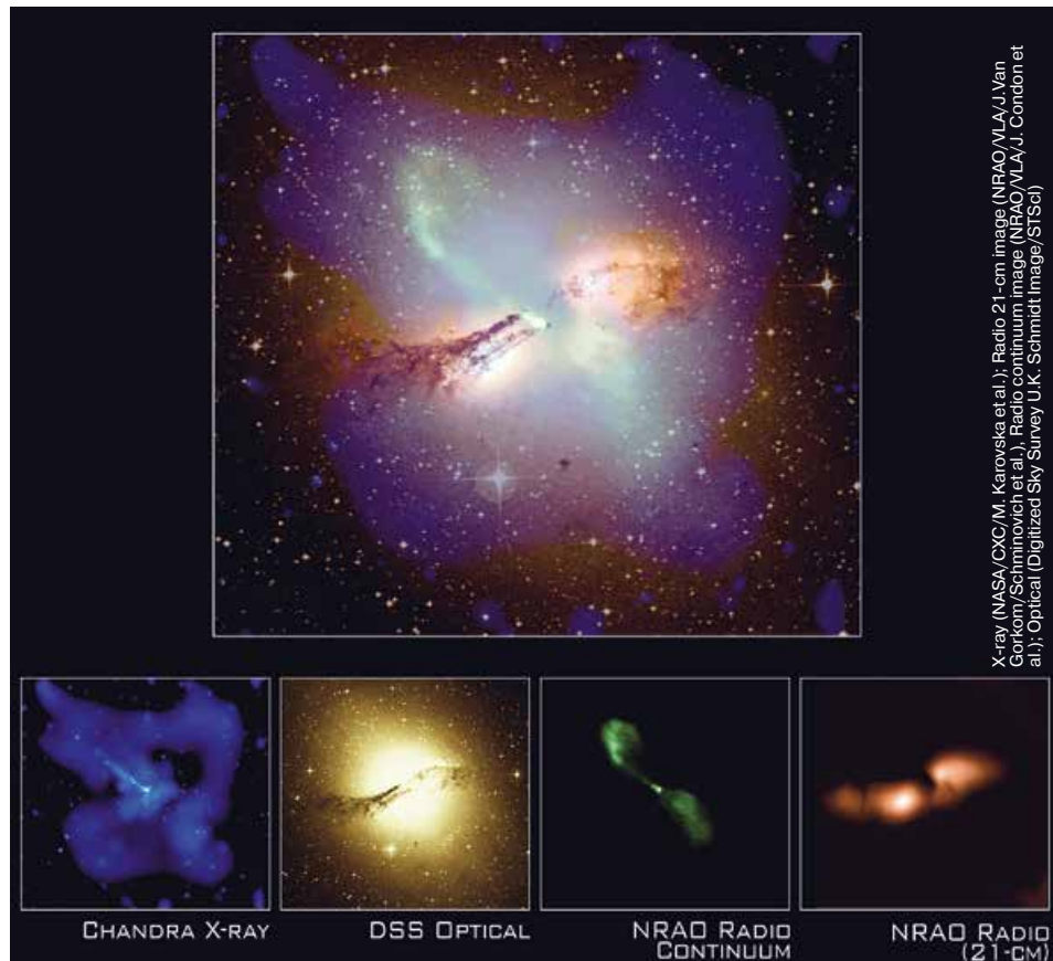
▲ Центавр А — ближайшая галактика с активным ядром.
