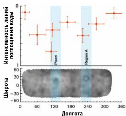
▲ Распределение источников водного пара на Церере. Изменение интенсивности линий поглощения водяного пара в спектрах Цереры по данным инфракрасной космической обсерватории Herschel (ESA). Наибольшая интенсивность соотносится с двумя темными регионами поверхности, названными Пиацци (Piazz) и Регион А — они были обнаружены в ходе наблюдений с помощью наземного телескопа Кекс II на Гавайских островах.
