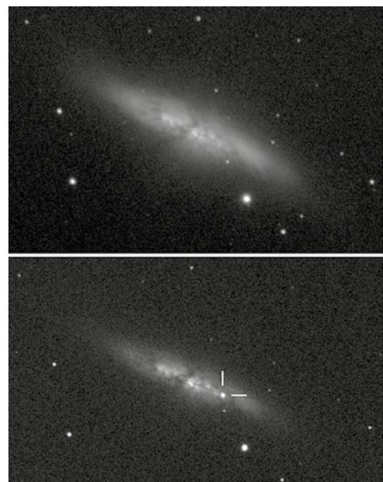
▲ Фотографии галактики М82, сделанные на обсерватории Лондонского университета до и после вспышки Сверхновой — 10 декабря 2013 г. и 21 января 2014 г.
