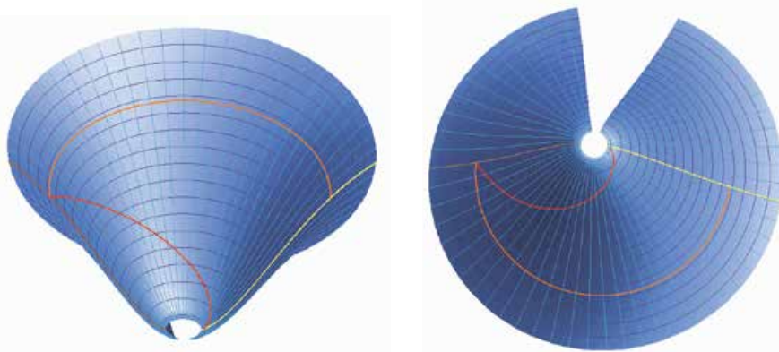
▲ Два вида условной изометрической проекции части наблюдаемой Вселенной, показывающие, как луч света (красная линия) может преодолеть эффективное расстояние в 28 млрд световых лет (оранжевая линия) всего за 13 млрд лет космогонического времени.
