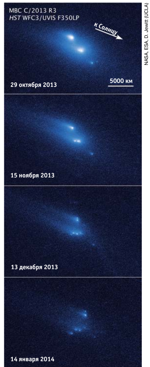
▲ Серия снимков, сделанных космическим телескопом Hubble, демонстрирует процесс распада астероида в течение нескольких месяцев в конце 2013 г.
