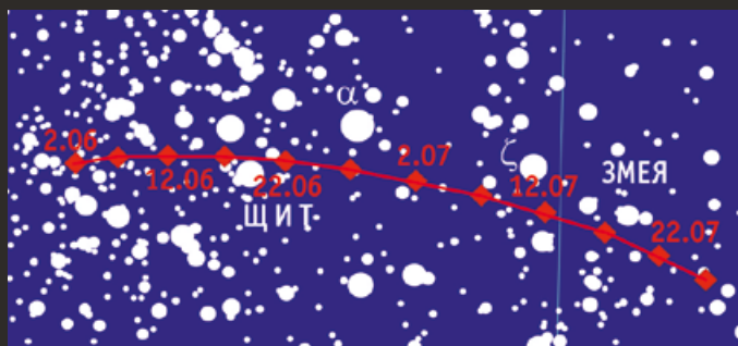
Видимый путь астероида Летиция в июне-августе 2014 г.
