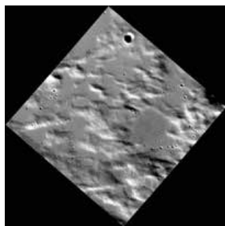
▲ Меркурианская поверхность с разрешением 7 м на пиксель.
