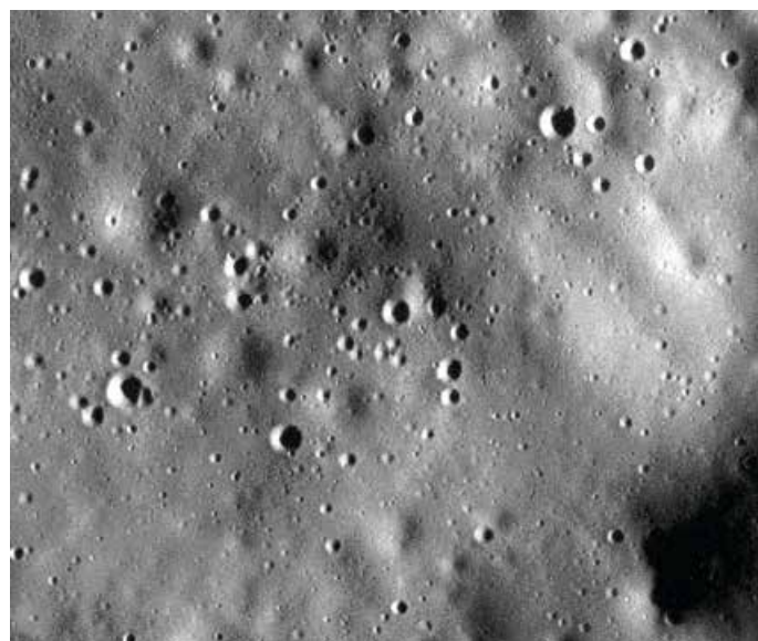
▲ Один из снимков поверхности Меркурия с рекордно высоким пространственным разрешением — до 5 м на пиксель.
