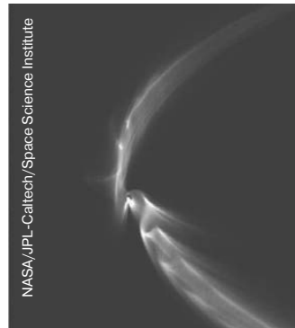
▲ Пылевые структуры, сформированные выбросами гейзеров у южного полюса Энцелада (показан результат компьютерного моделирования, практически полностью соответствующий наблюдательным данным).
