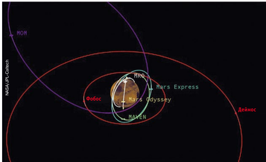
▲ На этой схеме показаны формы орбит и расстояния от поверхности Марса для пяти активных исследовательских аппаратов и двух его естественных спутников. Хорошо заметна возросшая вероятность взаимных столкновений (особенно в случае космического аппарата MAVEN)
