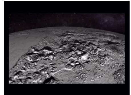
▼ Горная страна Норгей у южной границы Равнины Спутника.
