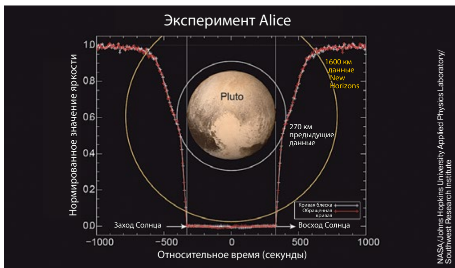
▲ Незадолго до вхождения зонда New Horizons в тень Плутона прибор Alice начал измерения видимой яркости Солнца. Она стала постепенно падать примерно за 5 минут до того, как светило скрылось за плутонианским диском. Вначале в основном регистрировалось поглощение солнечных лучей молекулярным азотом ( N_2 ), но по мере «захода» все четче проявлялись линии поглощения метана и более сложных углеводородов. Потом Солнце полностью «погасло». После его выхода из-за Плутона все атмосферные эффекты повторились практически идентично, только в обратном порядке.
