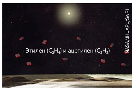
▲ Незадолго до вхождения зонда New Horizons в тень Плутона прибор Alice начал измерения видимой яркости Солнца. Она стала постепенно падать примерно за 5 минут до того, как светило скрылось за плутонианским диском. Вначале в основном регистрировалось поглощение солнечных лучей молекулярным азотом ( N_2 ), но по мере «захода» все четче проявлялись линии поглощения метана и более сложных углеводородов. Потом Солнце полностью «погасло». После его выхода из-за Плутона все атмосферные эффекты повторились практически идентично, только в обратном порядке.
