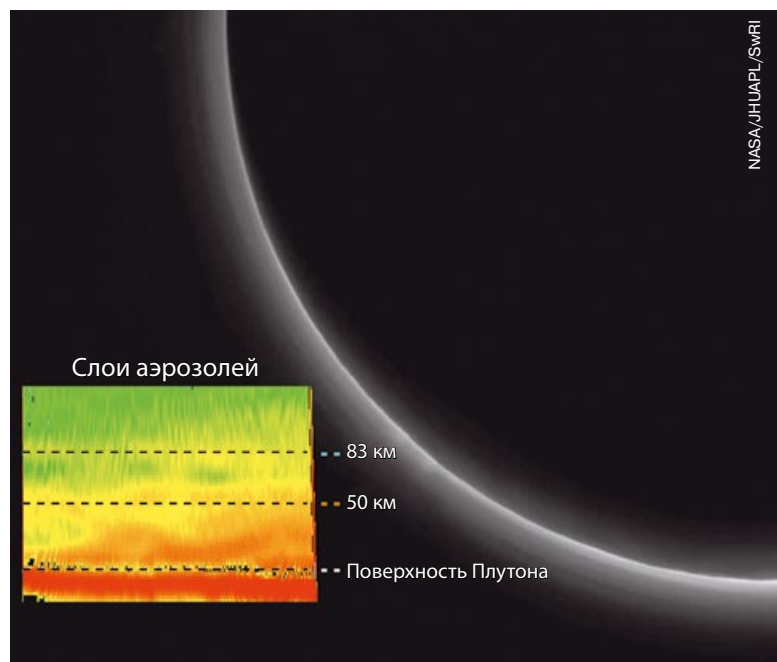
▲ Последний снимок Плутона космический аппарат New Horizons сделал из его тени, с расстояния около 2 млн км. На фотографии видна «плутонианская корона» — результат рассеяния солнечных лучей на частицах аэрозолей в атмосфере карликовой планеты. Большая толщина и высокая яркость светящегося ореола стала неожиданностью для ученых. Изображение было получено наземными приемными станциями 23 июля 2015 г. Север вверху.
