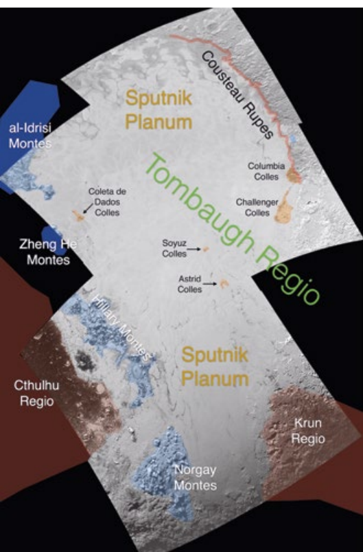
▲ Неформальные названия регионов Плутона и других деталей его поверхности, используемые сотрудниками группы сопровождения New Horizons, но пока не утвержденные официально. Часть имен была предложена в ходе интернет-кампании «Наш Плутон» (Our Pluto).
