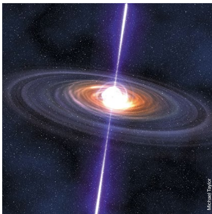
▲ Пульсар в представлении художника.
