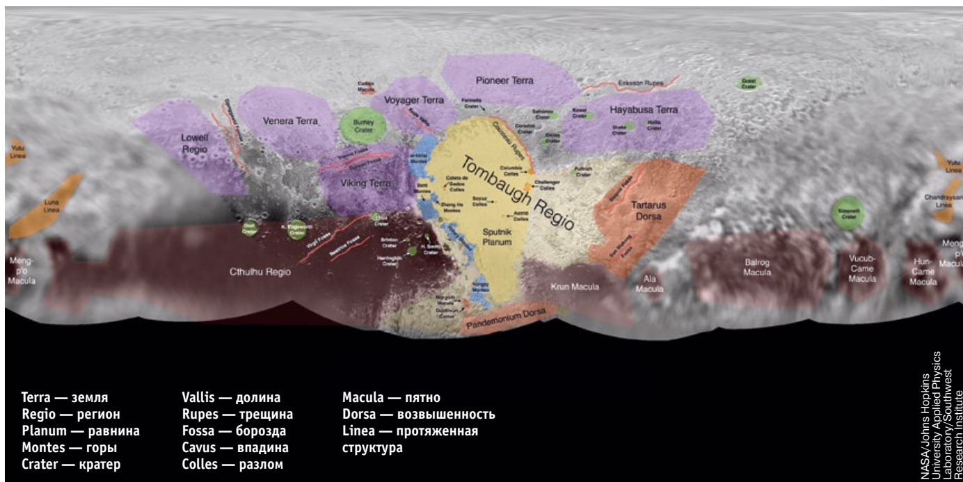
▲ Неформальные названия регионов Плутона и других деталей его поверхности, используемые сотрудниками группы сопровождения New Horizons, но пока не утвержденные официально. Часть имен была предложена в ходе интернет-кампании «Наш Плутон» (Our Pluto).
