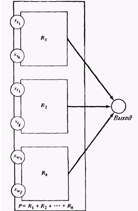
Рис. 12. Сеть Петри, слабо вычисляющая P(x_1, x_2, \dots, x_n) путей использования набора подсетей вида, изображенного на рис. 11.
