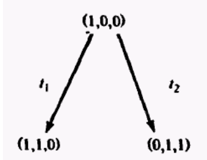
Рис. 10. Первый шаг построения дерева достижимости.
