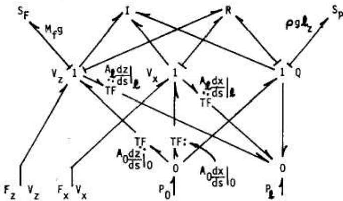
б. Граф связей
