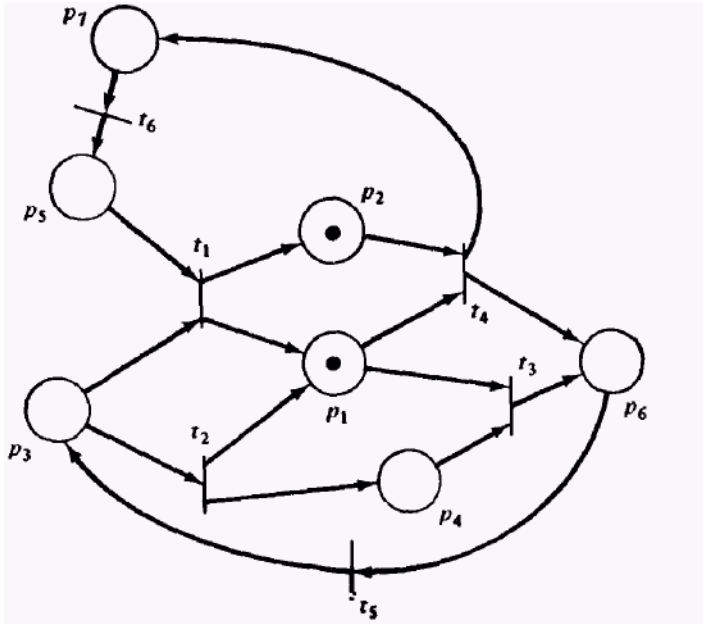
Рис. 6. Сеть Петри с областью ограничения \{p_3, p_7\} , которая означает, что в произвольной достижимой маркировке фишки могут быть либо в p_3 , либо в p_7 , но не в обеих одновременно.
