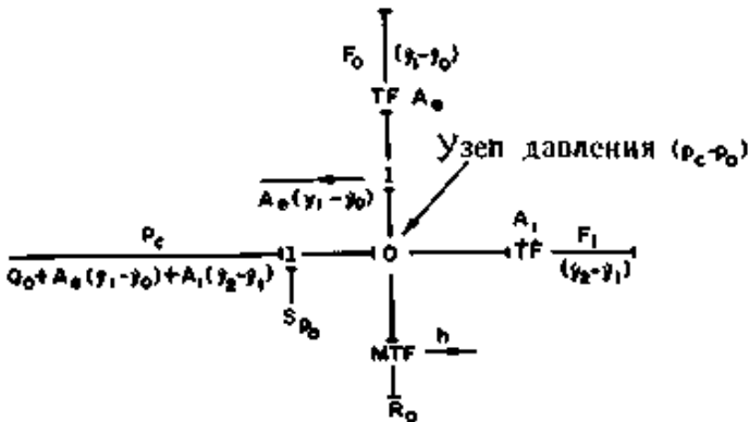
б. Гидромеханическое преобразование и утечки
