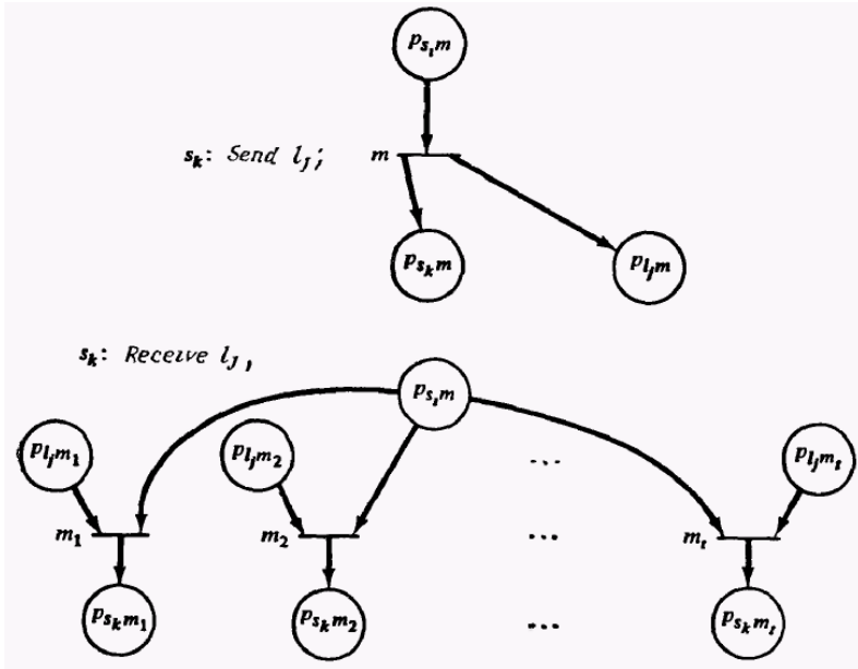
Рис. 10. Преобразование предложений send и receive в переходы сети Петри вверху — модель предложения s_k send с сообщением типа m в буфере сообщений. Канальный процесс — l_j , внизу — модель предложения s_k receive из канального процесса l_i . Возможные типы сообщения в l_i = m_1, m_2, \dots, m_t
