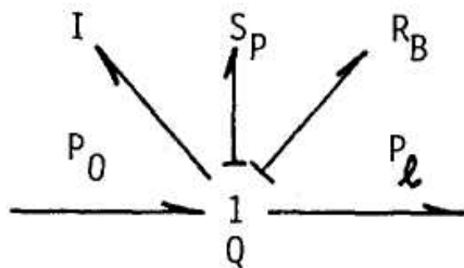
б. Граф связей
