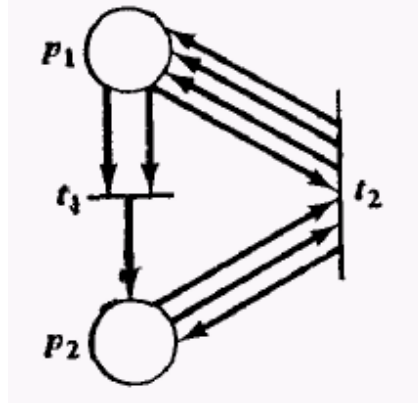
Рис. 7. Сеть Петри, иллюстрирующая пассивные маркировки для t_3 .
