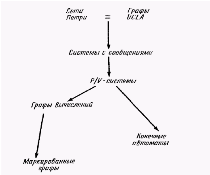
Рис. 18. Добавление графов UCLA к иерархии моделей.
