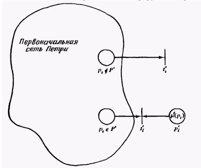
Рис. 2. Сеть Петри, служащая для доказательства сводимости задачи достижимости подмаркировки к задаче достижимости нуля. Подмножество позиций P' будет иметь маркировку \mu' в первоначальной сети тогда и только тогда, когда в модифицированной показанным здесь способом сети будет достижима нулевая маркировка.
