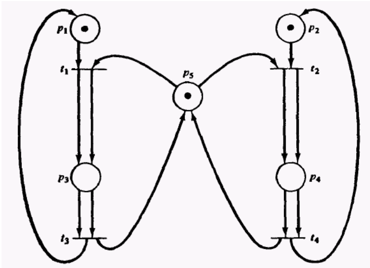
Рис. 4. Строго сохраняющая сеть Петри, эквивалентная сети, изображенной на рис. 3.
