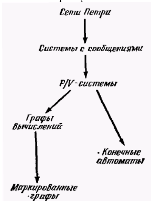
Рис. 13. Добавление систем с сообщениями к иерархии моделей.
