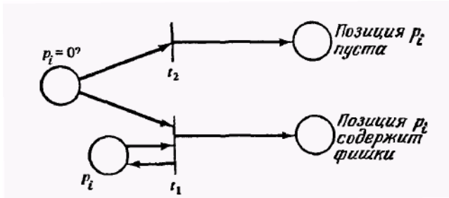
Рис. 11. Использование приоритетов для проверки позиций p на нуль. Переход t_1 имеет по сравнению с t_2 более высокий приоритет.
