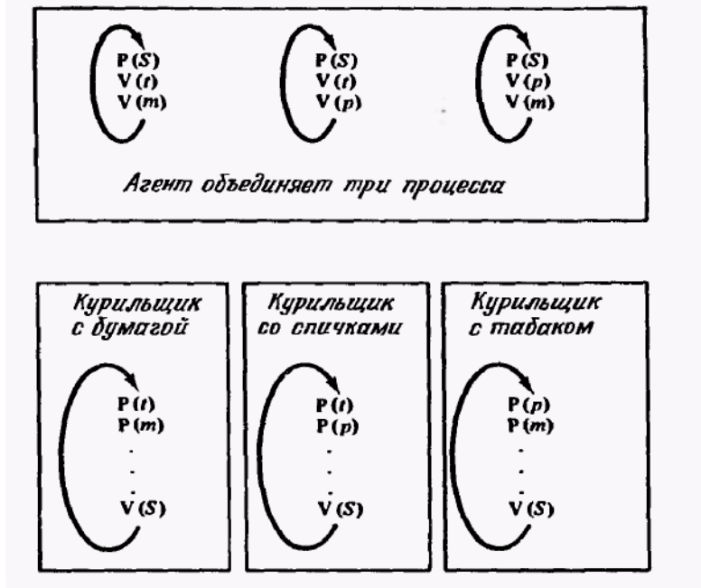
Рис. 3. Задача о курильщиках сигарет.
