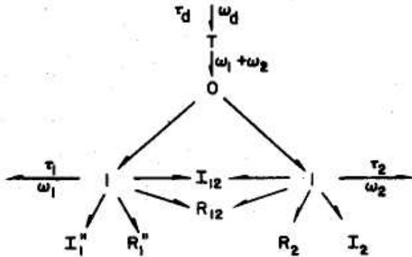
Рис.8. Граф связей дифференциала (рис.7).
