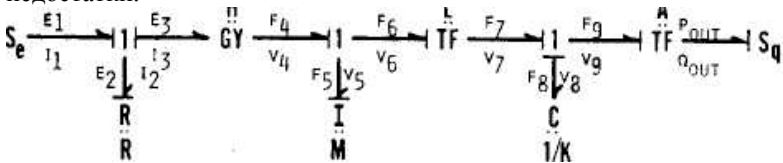
Рис. 8. Граф связей для модели Д с источником потока.
