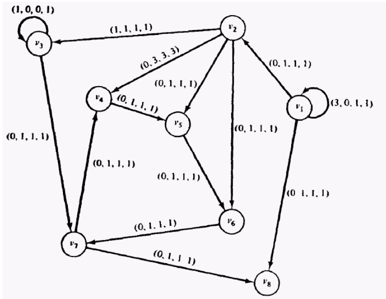
Рис. 2. Граф вычислений.
