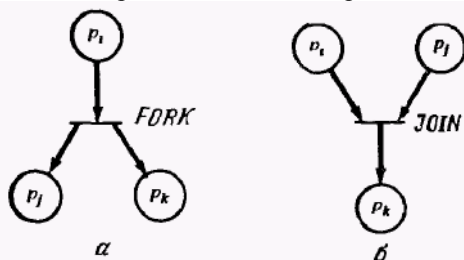
Рис. 26. Моделирование операций FORK и JOIN сетью Петри.
