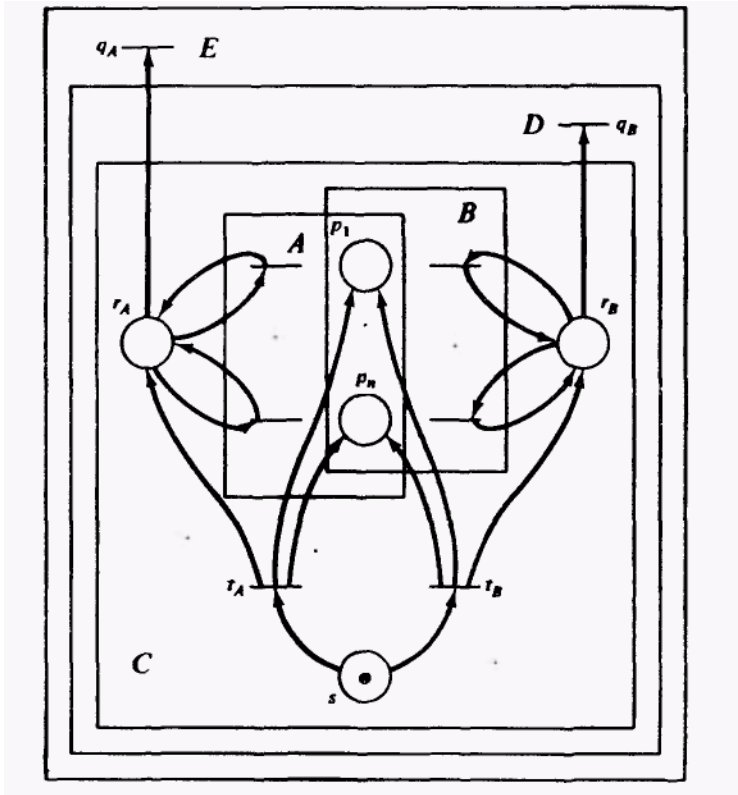
Рис. 14. Построение сетей Петри C , D и E из A и B , используемое для доказательства сводимости задачи подмножества для множеств достижимости к задаче равенства.
