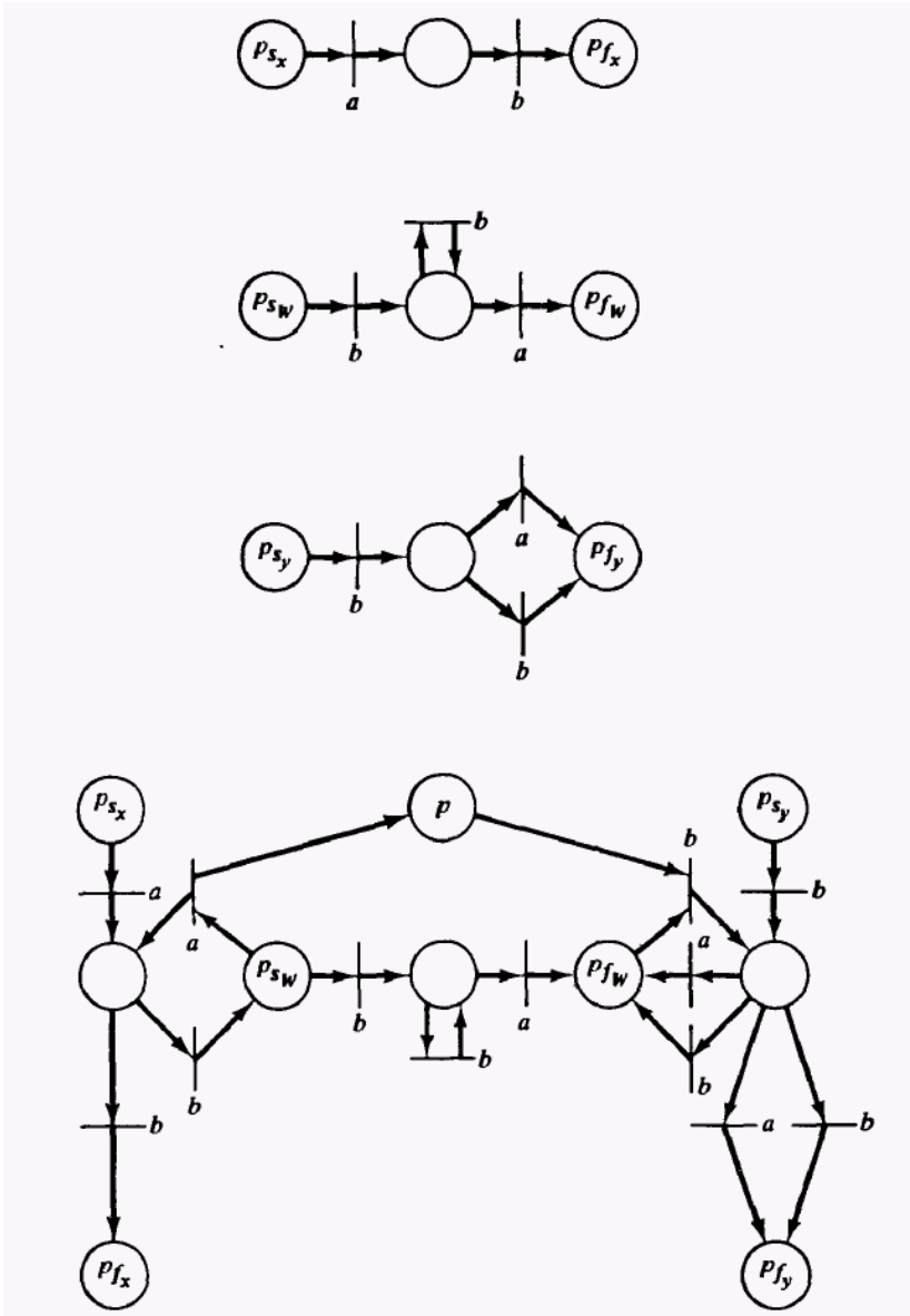
Рис. 14. Сеть Петри, порождающая язык \{x^i W y^j \mid i \geq 0\} . Эта конструкция показывает, что все ограниченные контекстно-свободные языки являются также языками сетей Петри.
