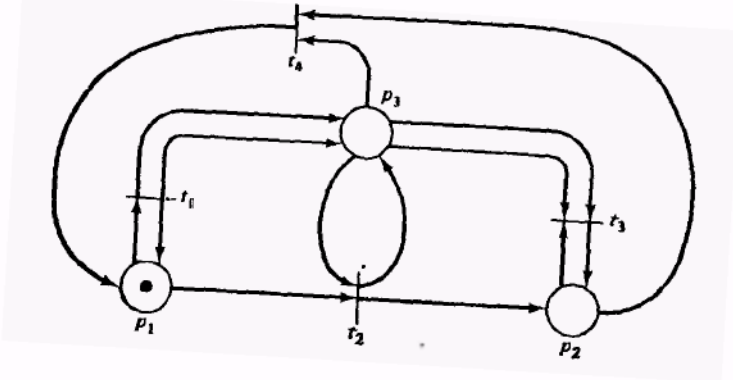
Рис. 23. Сеть Петри с возможным тупиком.
