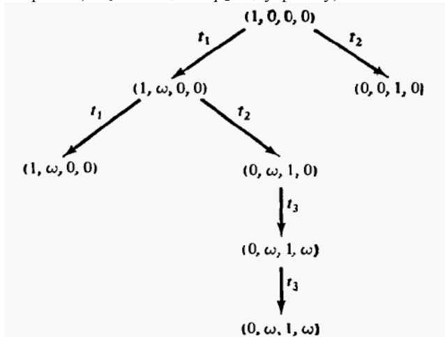
Рис. 19. Дерево достижимости для сети Петри, приведенной на рис. 18.
