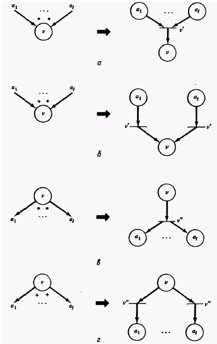
Рис. 16. Преобразование частей графа UCLA в сети Петри.
