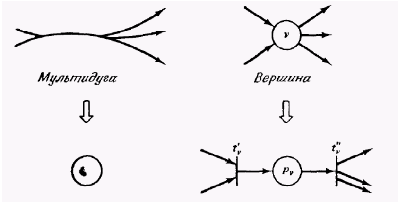
Рис. 15. Представление основных элементов графа UCLA в сети Петри.
