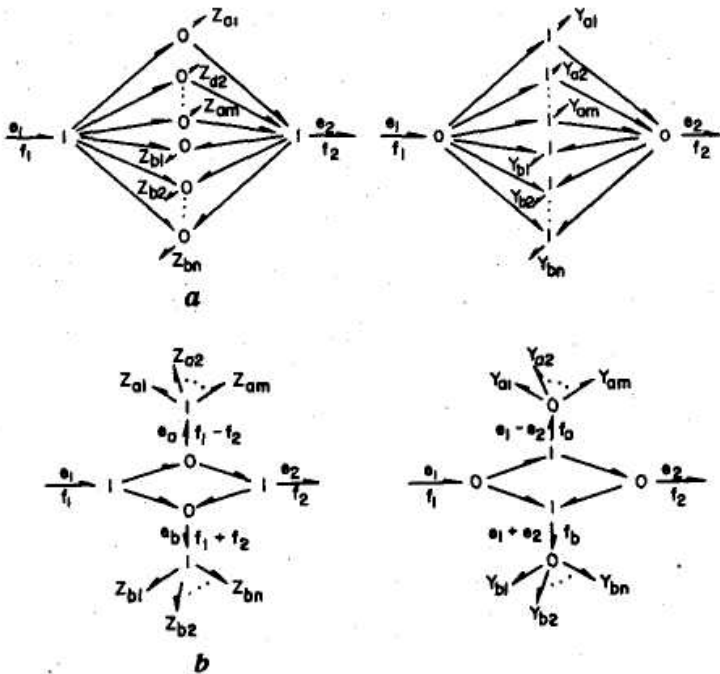
Рис.6. Сокращение простых сетей графов связей.
