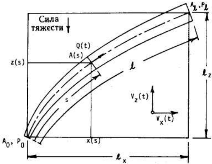
а. Схема системы
