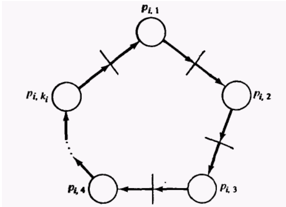
Рис. 4. Кольцо позиций, используемое в простой сети Петри для представления позиции обычной сети Петри. Число k_i позиций, представляющих позицию p_i , определяется максимумом сумм кратностей позиции.
