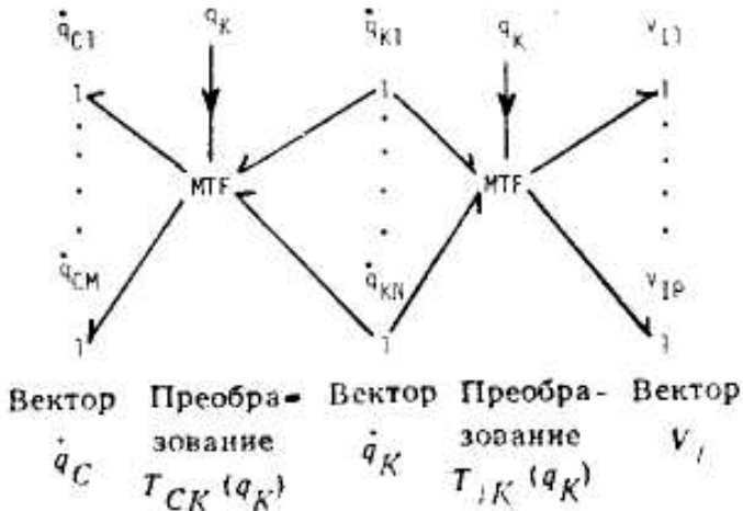
Рис.4. Символическая структура узлов, представляющая связи системы
