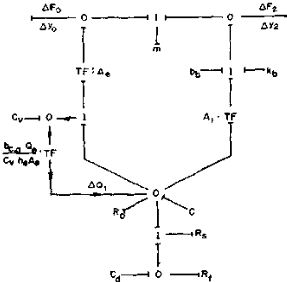
Рис. 6. Граф связей для линейной модели подвески
