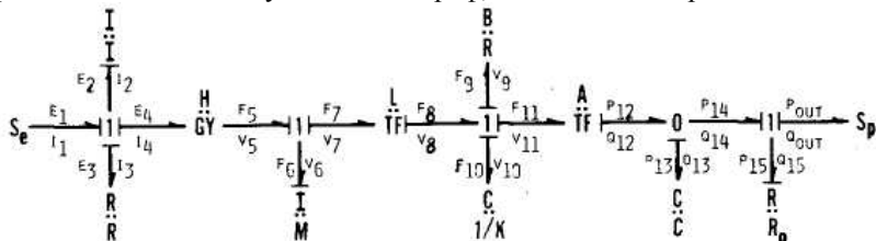
Рис. 12. Граф связей для модели Г.
