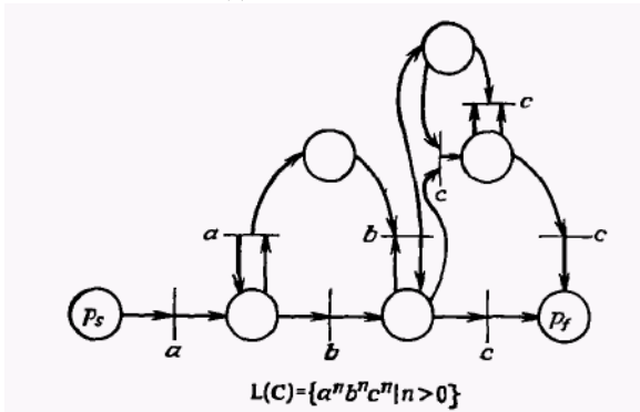
Рис. 13. Контекстно-связанный язык сети Петри, не являющийся контекстно-свободным.
