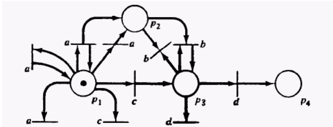
Рис. 3. Сеть Петри, язык L-типа которой совпадает с языком C-типа сети Петри, приведенной на рис. 2.
