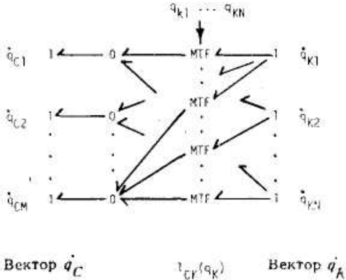
Рис. 2. Структура узлов, представляющая преобразование кинематических скоростей
