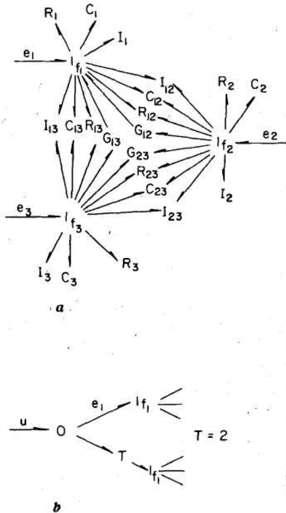
Рис.3. Альтернативный лагранжев граф связей для системы с тремя степенями свободы. a — общая форма без полной структуры входа; b — пример структуры входа.
