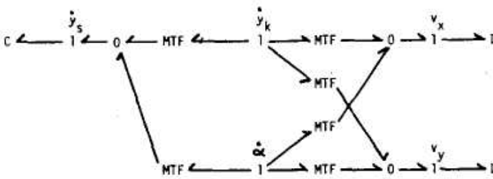
Рис.7. Модель графа связей колебательного звена из массы и пружины. a — совокупность ключевых геометрических переменных; b — подстановка преобразований T_{CK} и T_{IK} ; c - граф связей полной системы.
