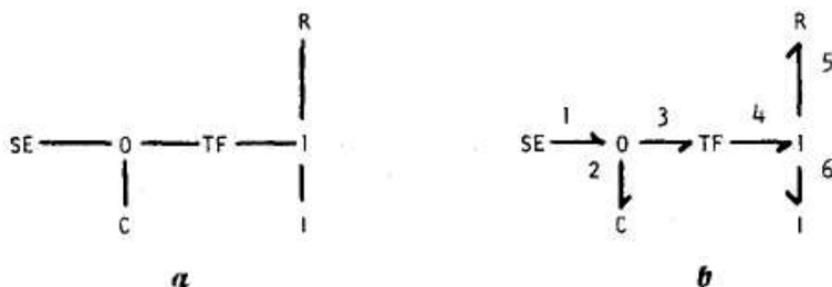
Рис. 2. Пример графа связей.
