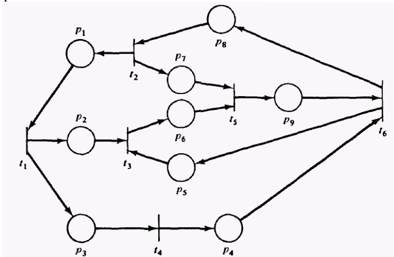
Рис. 6. Граф сети Петри, эквивалентный структуре, показанной на рис. 3.
