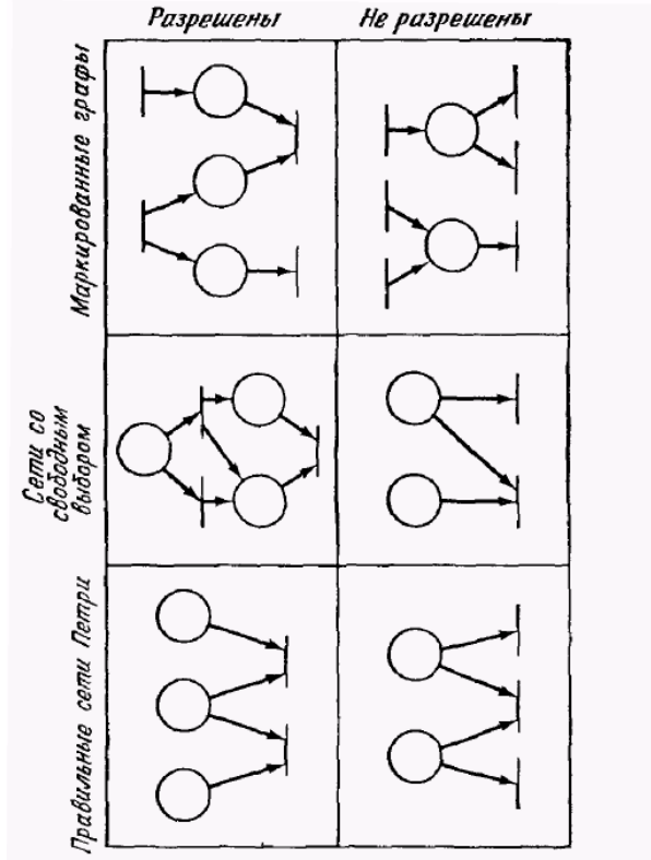
Рис. 14. Диаграмма осуществимости некоторых структурных конфигураций в различных сетях Петри.
