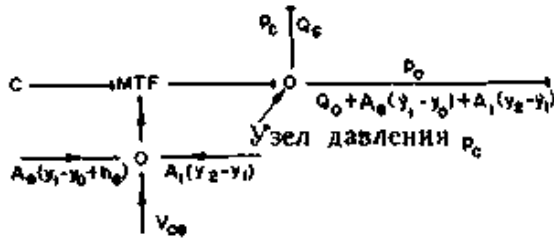
а. Соотношения для камеры сжатия
