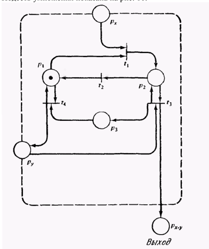
Рис. 10. Подсеть умножителя. Эта подсеть слабо вычисляет произведение x и y .
