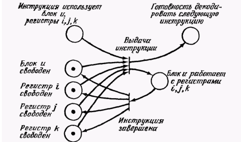
Рис. 20. Часть сети Петри, моделирующая устройство управления для ЭВМ, с кратными регистрами и кратными функциональными блоками.
