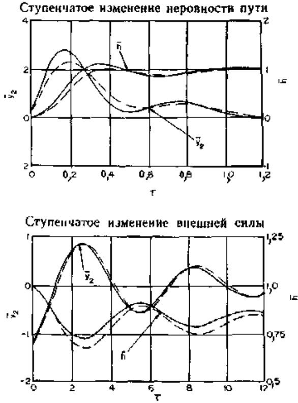
Рис. 10. Переходные характеристики конфигурации 3. f_n=2 Гц, h_e=1,27 см
