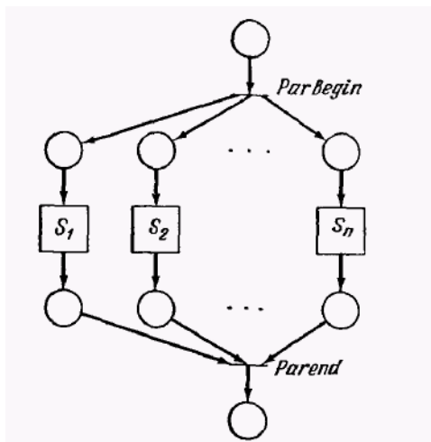
Рис. 27. Моделирование структуры parbegin S_1; S_2; \dots; S_n parend в сети Петри. Каждый квадрат есть представление сетью Петри утверждений S_1, S_2 и т. д. Здесь иллюстрируется также иерархическая природа моделирования сетями Петри.
