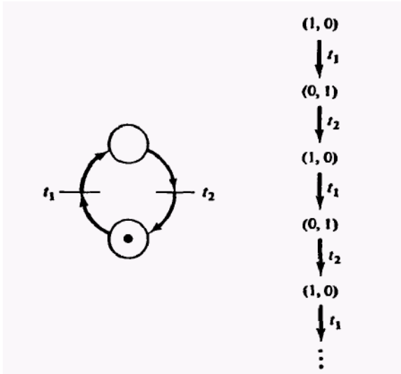
Рис. 13. Простая сеть Петри с бесконечным деревом достижимости.
