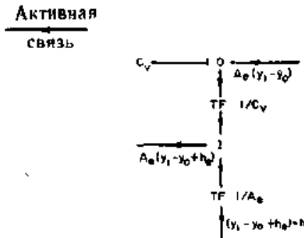
b. Активные связи для определения h
