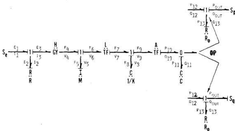
10. Граф связей для модели F.
