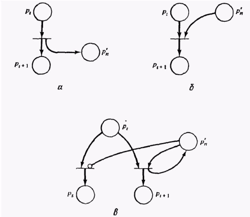
Рис. 12. Преобразование инструкции (номер i ) регистровой машины в переход расширенной сети Петри со сдерживающими дугами. a — P(n) : увеличить содержимое регистра n на 1; \delta — D(n) : уменьшить содержимое регистра n на 1 (содержимое регистра n должно быть положительным), \beta — J(n)[s] : переход к инструкции s в случае нулевого значения регистра n .
