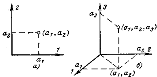
Рис. 1. Проекции двух- и трехэлементного кортежа.
