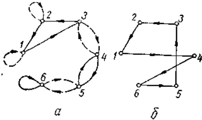
Рис. 8. Графы подстановок ( a ) и композиции подстановок ( б )
