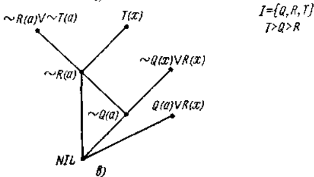
Рис. 12.2. Граф опровержения, полученный PI -резольвцией, положительной гиперрезольвцией и отрицательной гиперрезольвцией.
